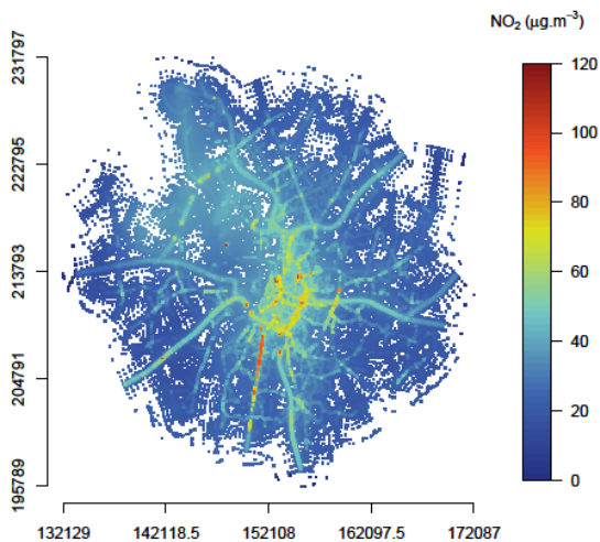
Moyennes annuelles NO 2 modélisées
